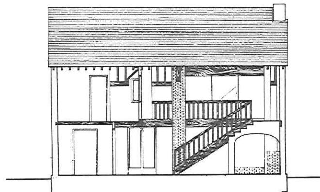
COUPE
